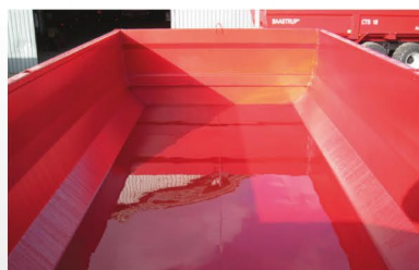
Den koniske kasse er lavet i Hardox 450. Bunden er lavet af to stykker, det er ingen tværgående svejsninger. Der er kun én langsgående svejsning, hvilket gør tipping lettere.
